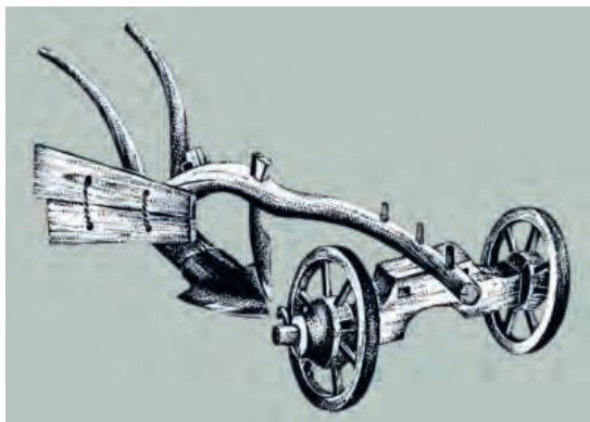
Булгарский плуг. Реконструкция Болгар сабаны. График реконструкция
