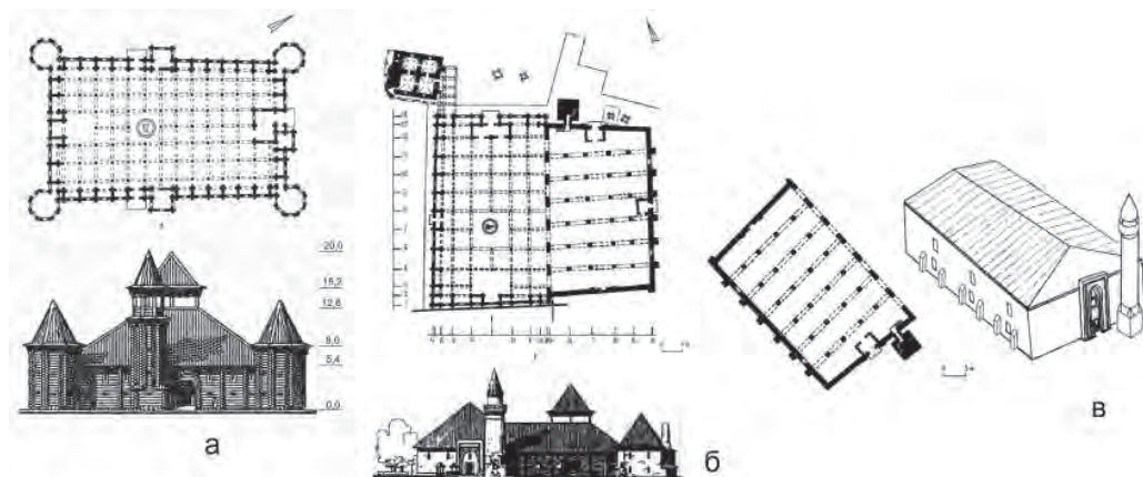
Варианты реконструкции Соборной мечети в Биляре (а,б – по С.С. Айдарову и Ф. Забировой; в – по Э.Д. Зеливинской)
