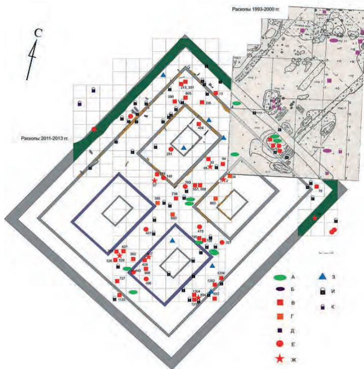
Центральный базар. План раскопок (по В.Ю. Ковалю и Д.Ю. Бадееву)
