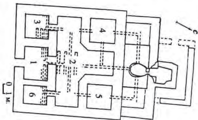
Баня № 3. Схема размещения внутренних помещений З нче мунча. Эчке бүлмәләренң урнашу тәртибе
