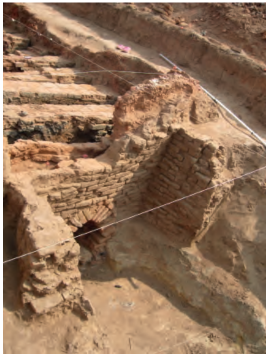
Горн для обжига кирпича Раскопки Селитренного городища. 2013
