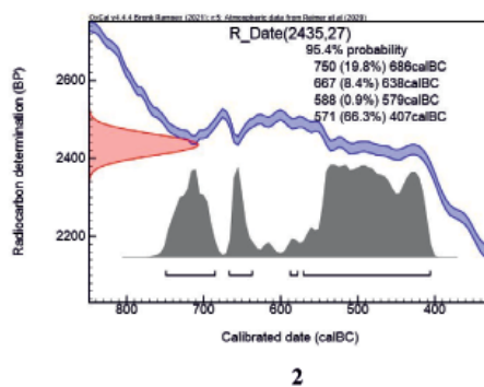
Рис. 3. Макарьевское городище. Данные радиоуглеродного анализа зёрен ячменя. 1 – образец S04; 2 – образец S05.
