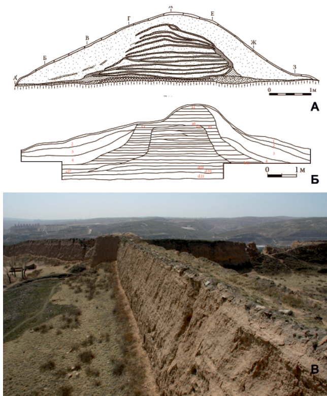
Рис. 2. Стены, выстроенные по китайскому методу ханту. А – разрез стены Джигитовского городища в Приморье (по: Дьякова, 2009, рис. 46). Б – разрез южной стены внутреннего города Балиньчэна в Северо-Восточном Китае (по: Стоякин и др., 2020, рис. 8: 2). В – частично руинированный отрезок Великой китайской стены, выстроенной по методу ханту близ г. Датун (из свободного интернет-ресурса. Адрес: https://maximus101.livejournal.com/42772.html . Дата обращения 11.07.2024).
