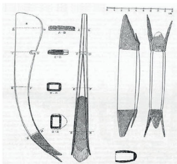
Рис. 5. Пластины лука аварского периода из Сегед-Фехертó А (Szeged-Fehértó A, Венгрия), погр. 26 и 32. На левой части рисунка стоит обратить внимание на рифление поверхности пластин. Склейка была усилена обвязкой. Справа, на рисунках поперечных сечений видны, что пластины окружают рога и рукоять лука (Balogh, 2016, 213).
