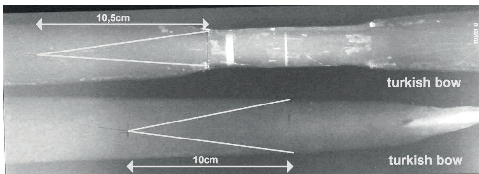
Рис. 8. Рентгеновский снимок рукояти и рога турецкого лука. Слева врубки рога и рукояти лука выделены толстой светлой линией. На правой верхней части снимка можно увидеть врубку рукояти в виде слабой V-образной формы без выделения. Этим лукам перевязка больше не требуется из-за врубных и клеенных соединений ( www.atarn.net ).
