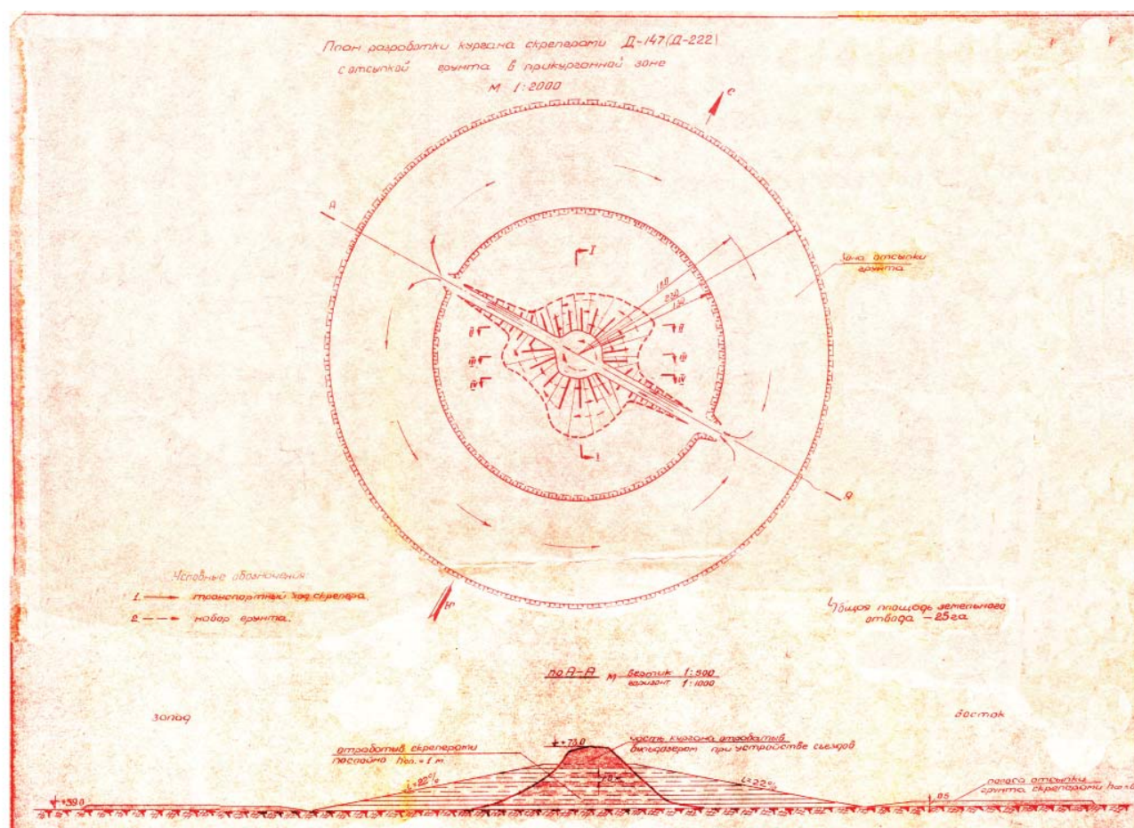
Рис. 7. Нечаева Могила. Схема движения скреперов и складирования вывезенного грунта при разработке насыпи кургана скреперами, а также схема устройства бульдозерных въездов на курган для скреперов. К проекту раскопок Нечаевой Могилы 1966 г. Из архива С.В. Полина.
