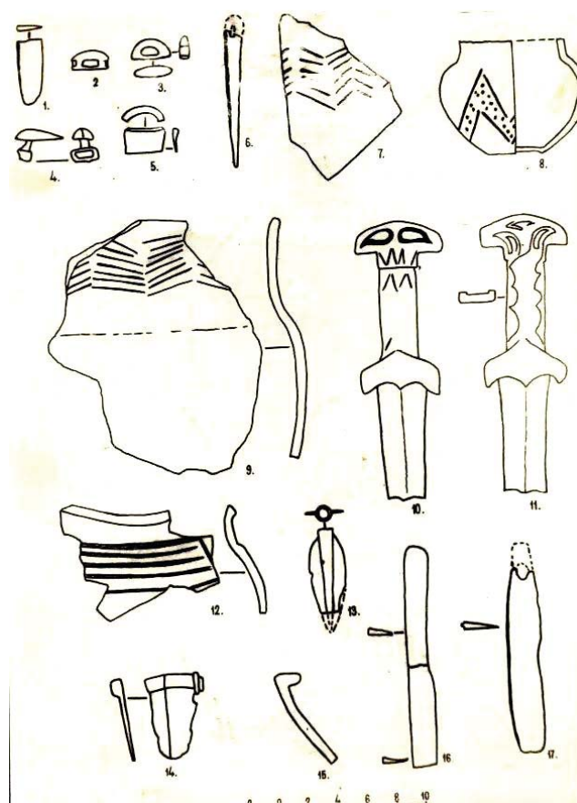
Рис. 10. Фото рисунков бронзовых изделий, собранных во время строительства Ташкентского канала (РЖВ). Fig. 10. Photos of drawings of bronze products collected during the construction of the Tashkent Canal (RZHEV).
