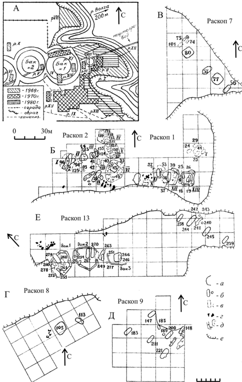
Рис. 8. План Тетюшского могильника. А – план памятника; Б – план раскопов 1 и 2; В – план раскопа 7; Г – план раскопа 8; Д – план раскопа 9; Е – план раскопа 13.
