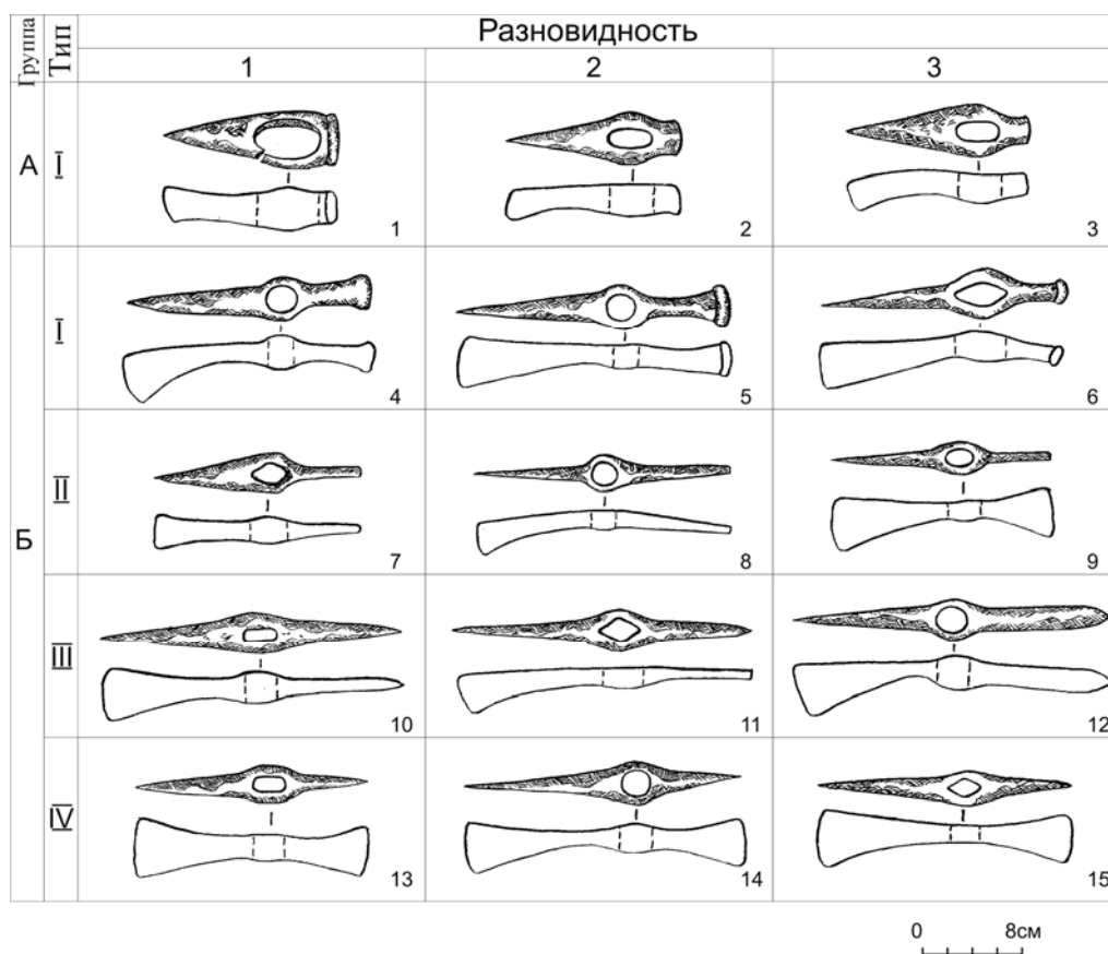
Рис. 29. Железные топоры Старшего Ахмыловского (2–6, 10–15) и Акозинского (1, 7–9) могильников: 1 – кв. О/01 раскопа 1971 г.; 2 – п. 835; 3 – кв. Ж/8 раскопа 1962 г.; 4 – п. 743; 5 – п. 336; 6 – п. 421; 7 – п. 73; 8, 9 – кв. Ю/7 и Я/8 раскопа 1971 г.; 10 – п. 908; 11 – кв. В/2 раскопа 1962 г.; 12 – п. 543; 13 – п. 808; 14 – п. 183; 15 – находка на усадьбе А. Ерофеева.
