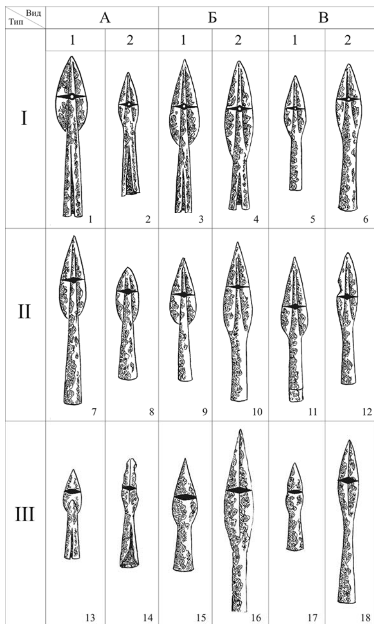
Рис. 22. Железные наконечники копий Старшего Ахмыловского могильника. Типологическая таблица (места находок указаны в табл. XIV; изделие типа I А происходит из кв. Е/8 раскопа 1958 г. из Аозино).
