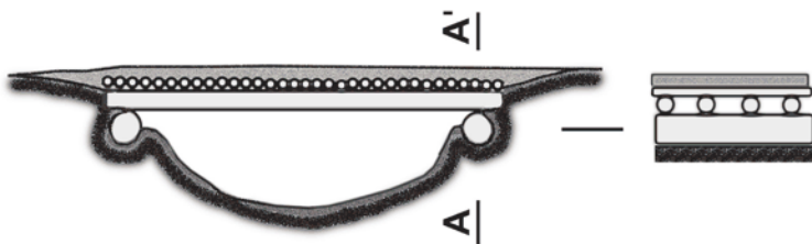
Рис. 39. Конструкция простого балочного моста сибирских татар (по Матвеев А.В., Татауров С.Ф., 2014).
