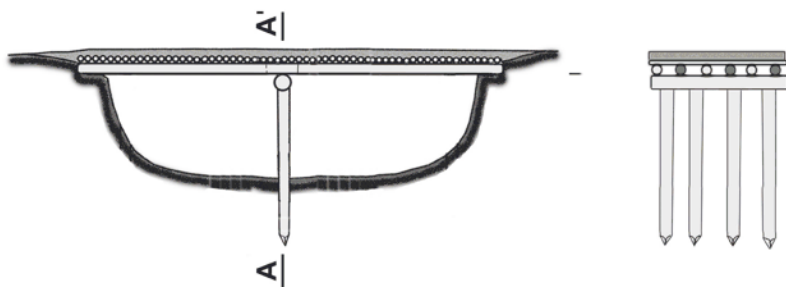
Рис.41. Конструкция свайного двухпролетного моста сибирских татар (по Матвеев А.В., Татауров С.Ф., 2014).
