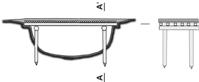
Рис. 40. Конструкция свайного моста сибирских татар (по Матвеев А.В., Татауров С.Ф., 2014).
