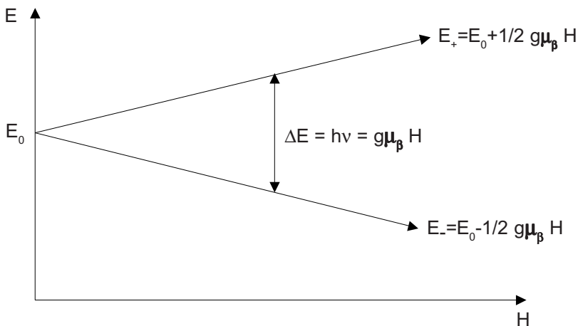
Рис.2. Зеемановское расщепление энергетических уровней
