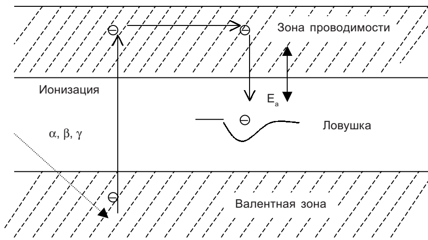
Рис. 8. Схема захвата электронов в минерале
