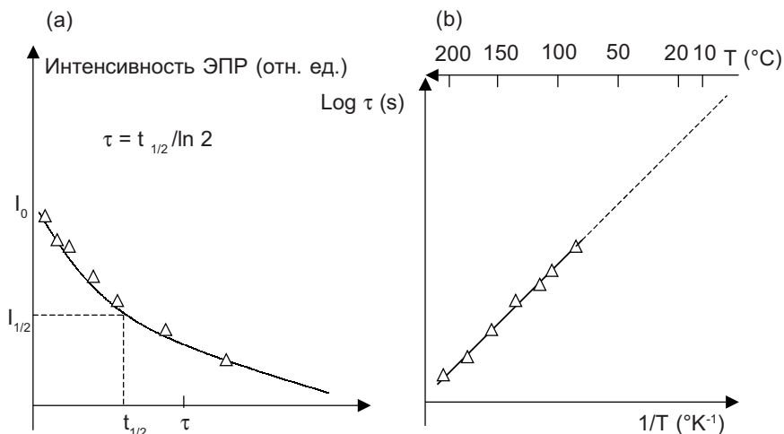
Рис. 13. Определение величины времени жизни \tau парамагнитного центра.
